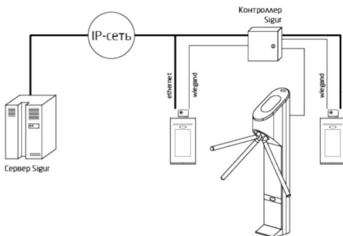
Структурная схема подключения терминала распознавания лиц Hikvision к СКУД Sigur.
