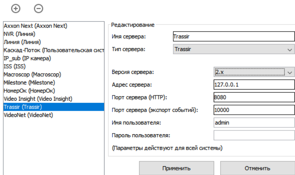
Настройка системы видеонаблюдения Trassir 2.
