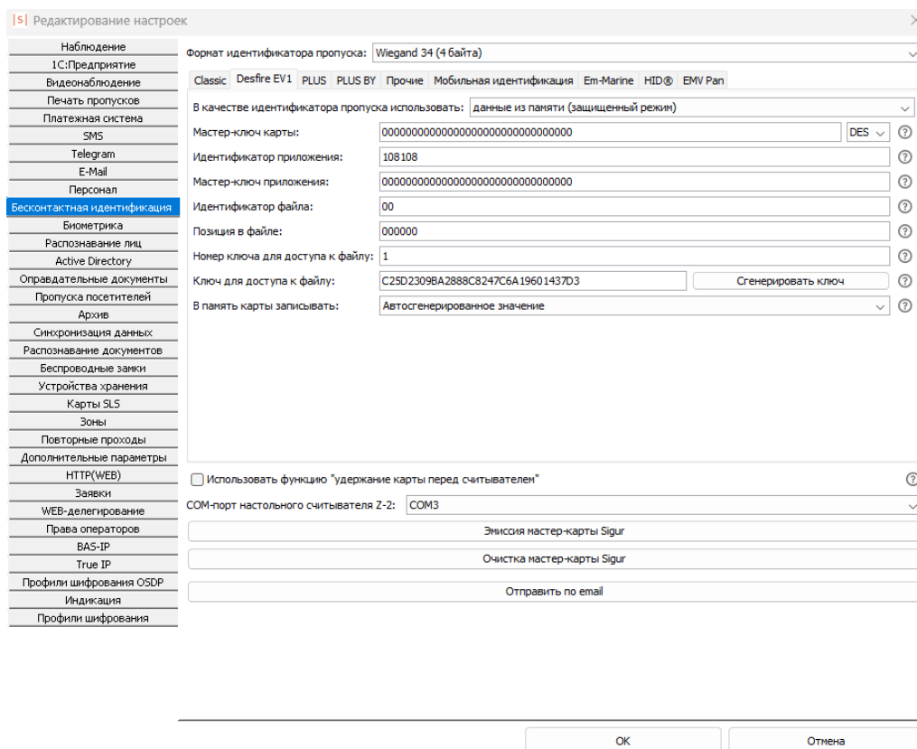
Окно настроек карт Mifare: пример корректных настроек для карт Mifare Desfire EV1.
