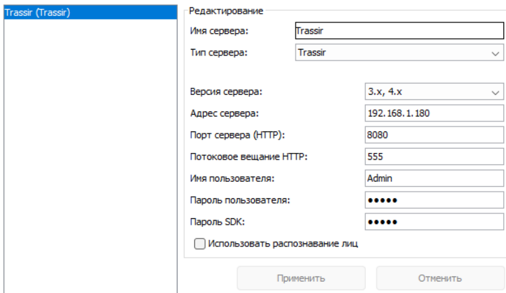
Настройки сервера системы видеонаблюдения Trassir 3 или 4.
