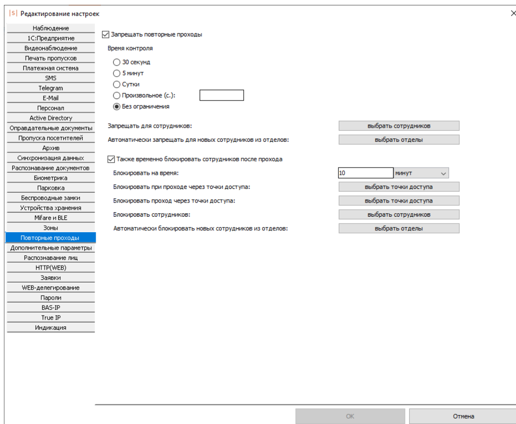
Вид вкладки «Повторные проходы».
