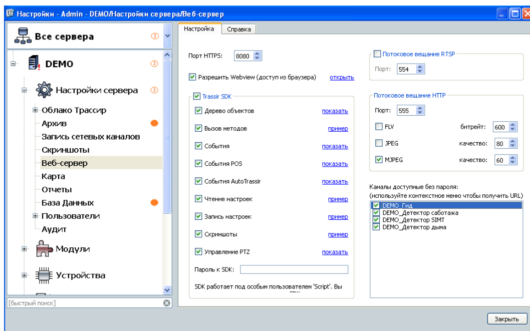
Настройки сервера системы видеонаблюдения Trassir 3.
