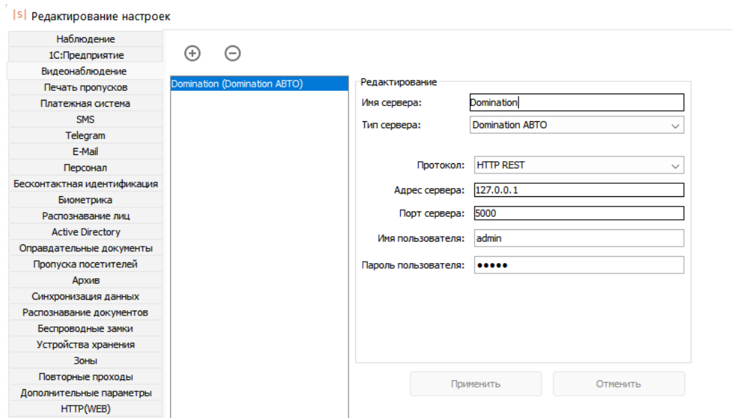
Настройки в Sigur для сервера видеоаналитики Domination.
