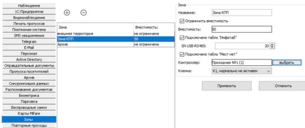
Интерфейс управления вместимостью зон.
