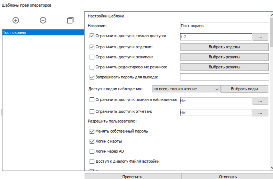
Шаблоны прав операторов.
