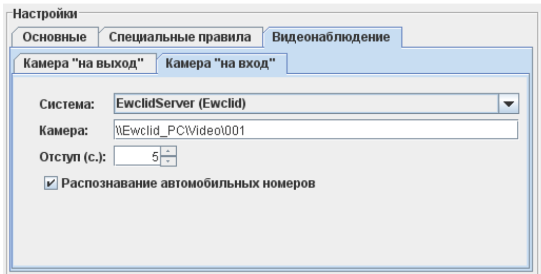
Пример назначения камеры Ewclid на вкладке «Оборудование».
